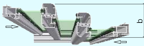
3-delat parti, b=94\text{mm} .
